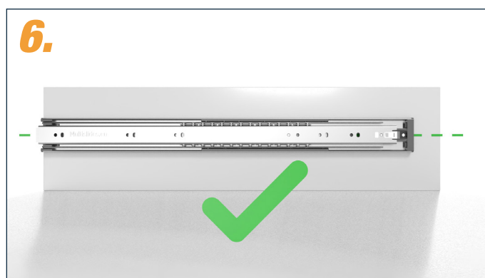
6. Les rails extérieurs doivent être parallèles au sol.
