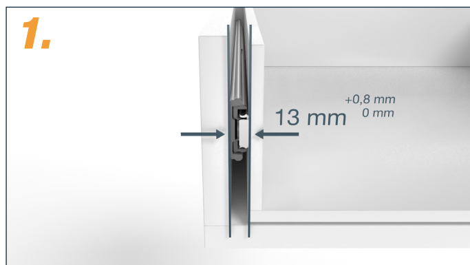
1. Distance minimale entre le caisson et le tiroir à respecter!
